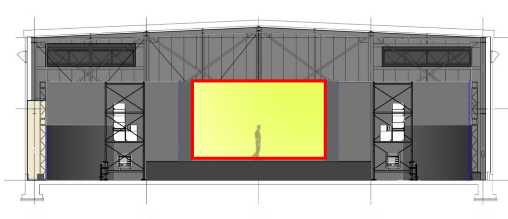
断面
